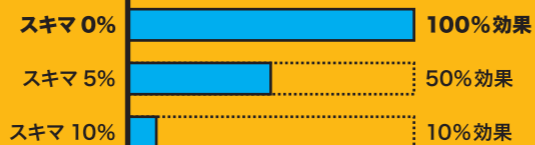
天井のスキマと断熱効果の関係...
