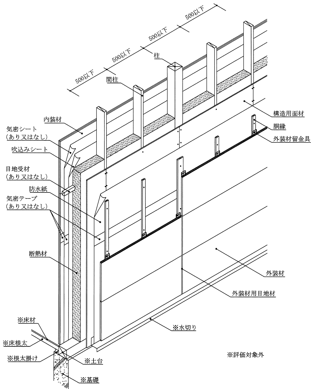
透視図
