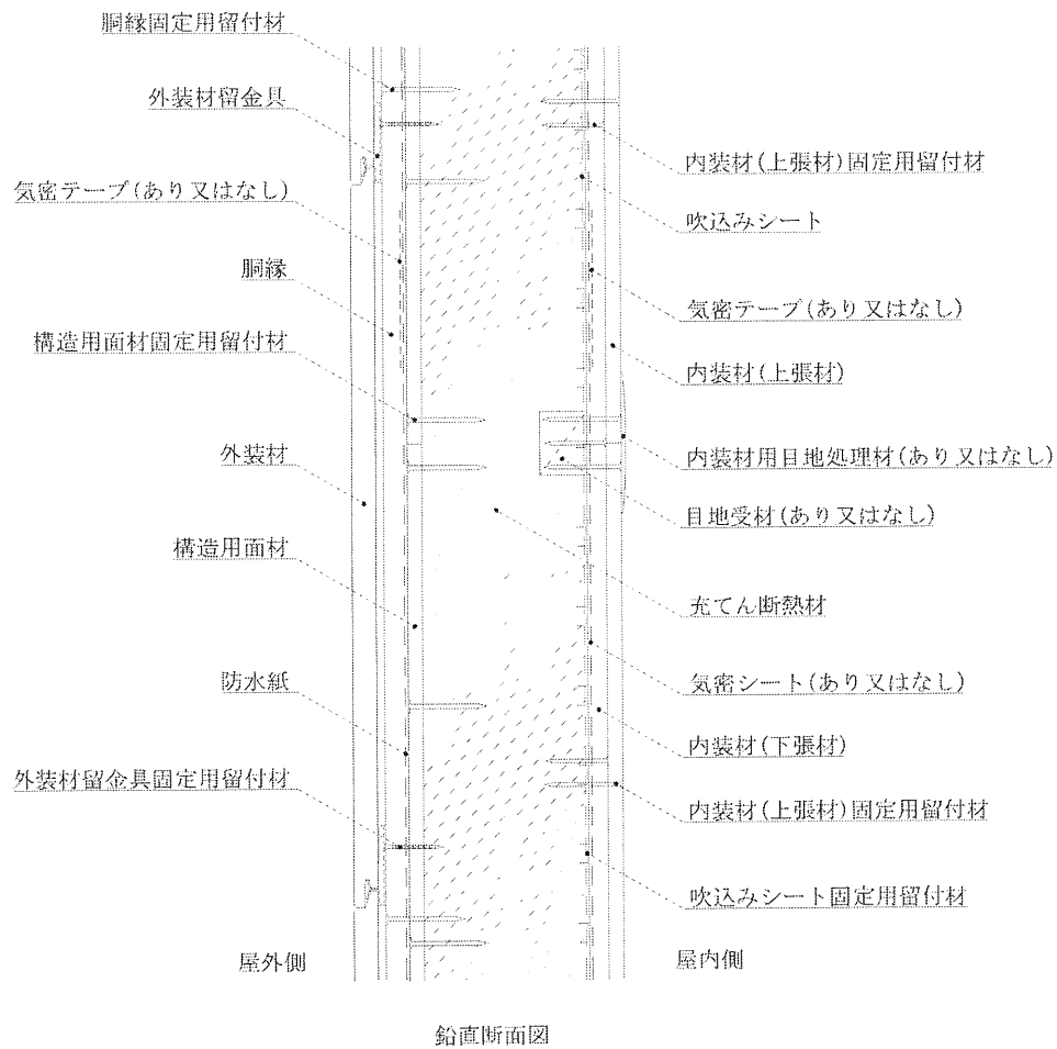
図2 構造説明図
