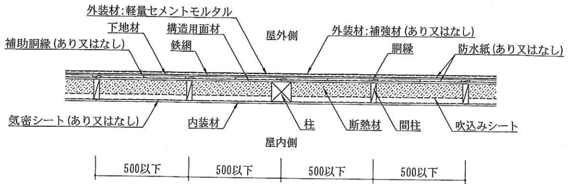
水平断面図 (通気仕様) (構造用面材あり・下地材あり仕様)
